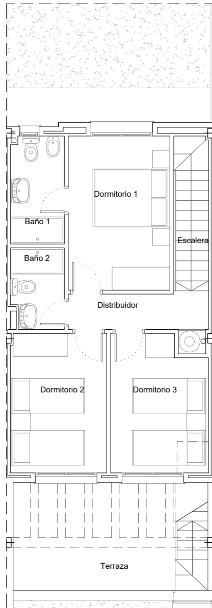
Planta Primera. 1:100
